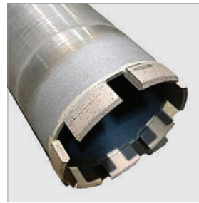
Напайка сегментов серебросодержащим припоем
