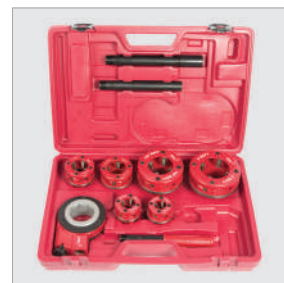
Комплект V-Cut 2" (№ 2.00013)
