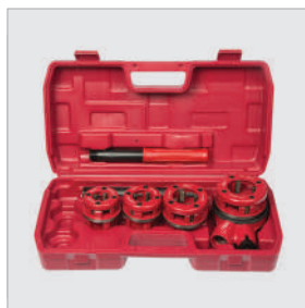
Комплект V-Cut 1/1/4" (№ 2.00012)
