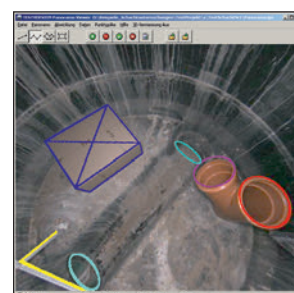
PANORAMO SI в качестве дополнения системы инспектирования
