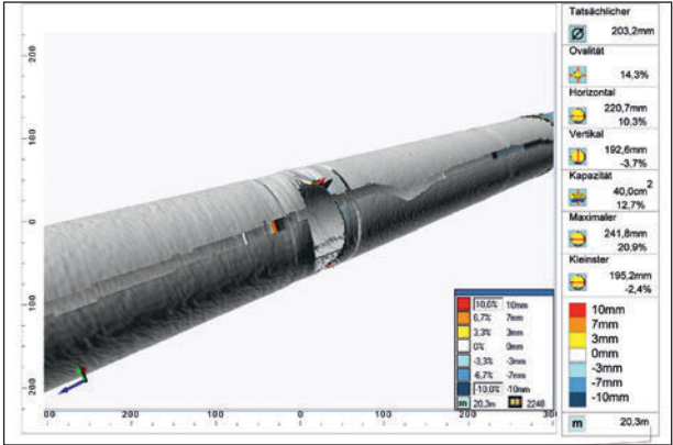
Графическое изображение замера овальности
