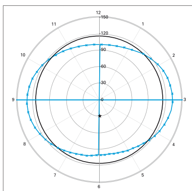
График деформации трубы
